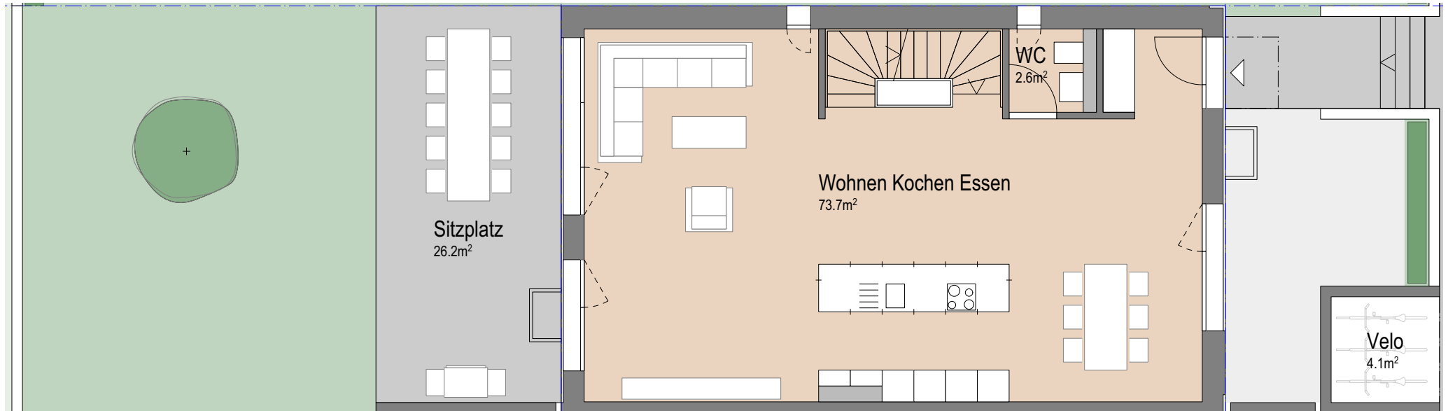
Erdgeschoss Variante Zweifrontenküche
