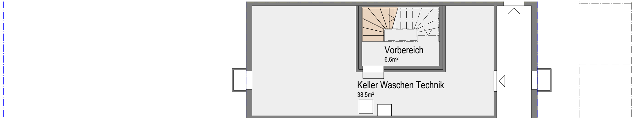
Untergeschoss Reiheneinfamilienhaus 6F
