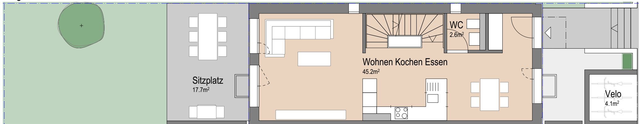
Erdgeschoss
